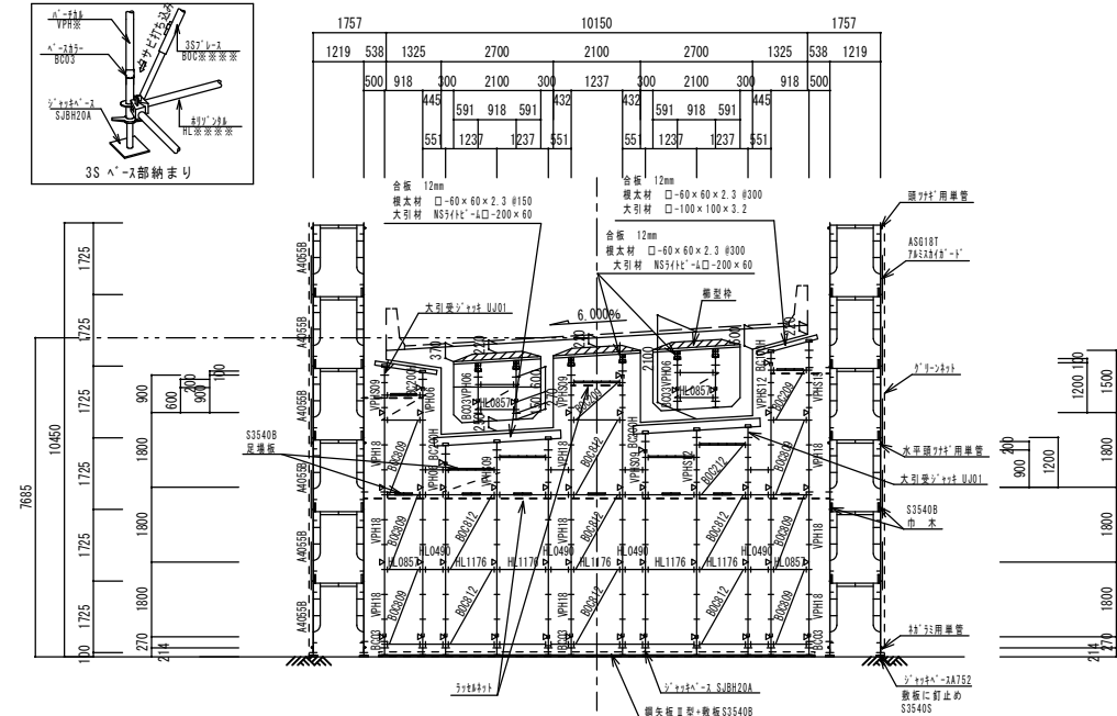
P4~A2断面図 S=1/100
