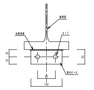
取付ベース詳細図
