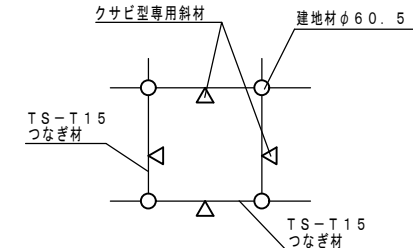
上部平面図 1/100
