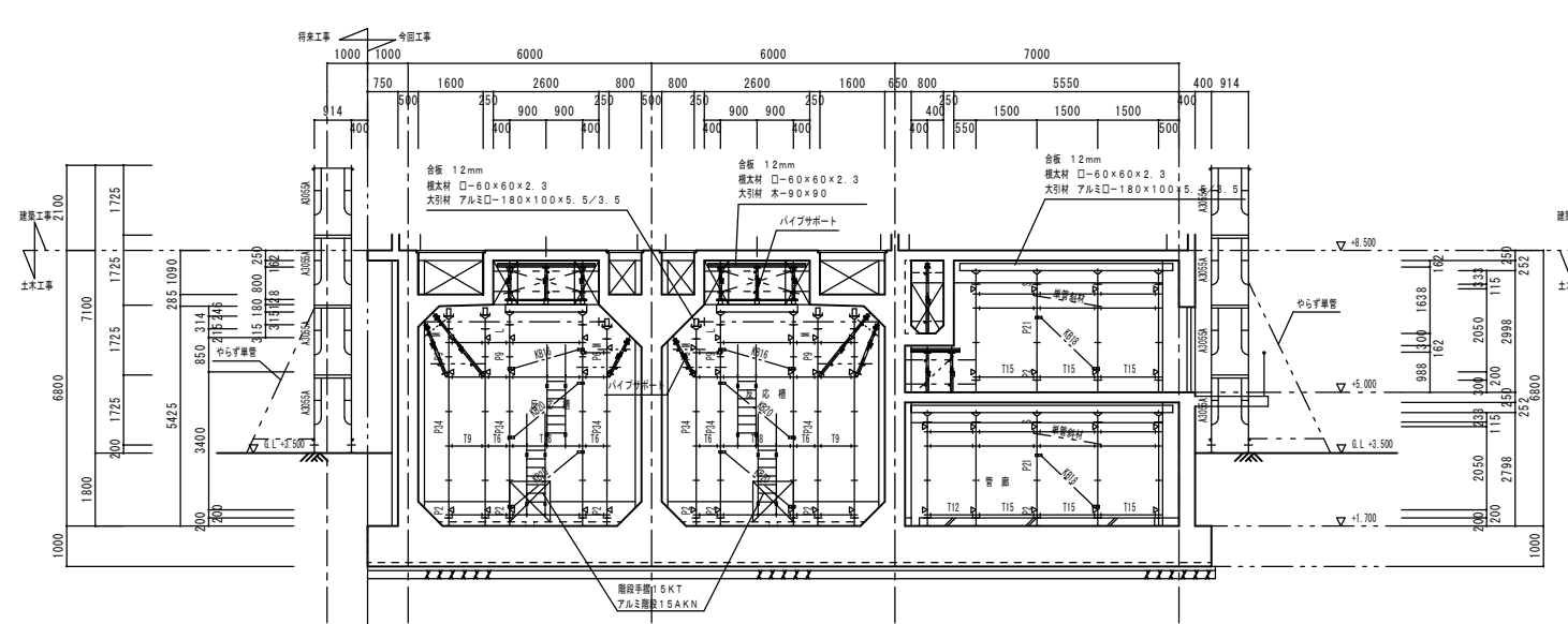
F-F 断面図 1/100
