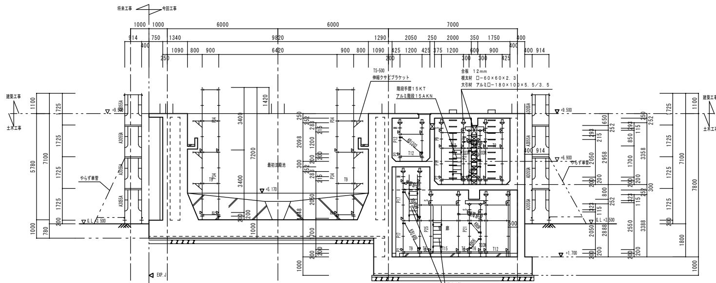
C-C 断面図 1/100
