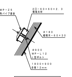
横端太+桟木 詳細図 1/10
