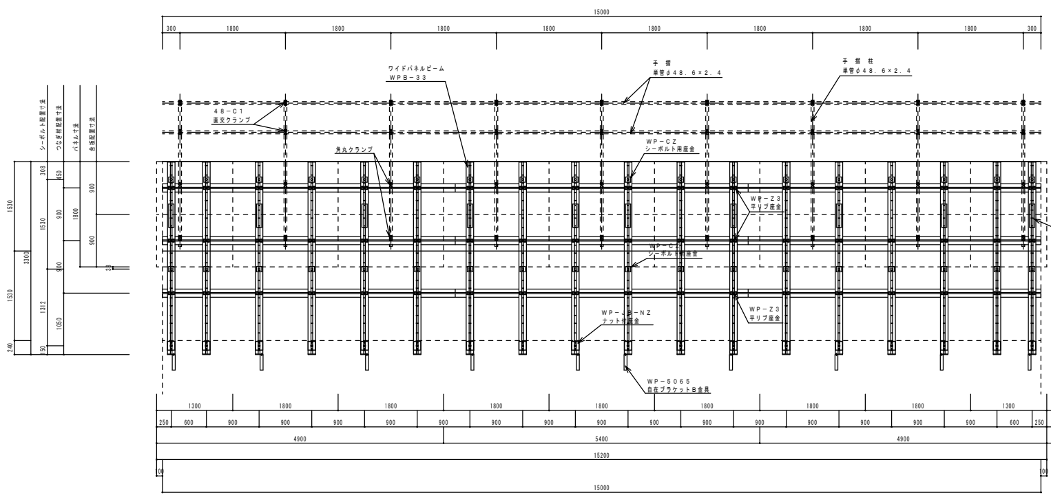
B 側面図 1/40
