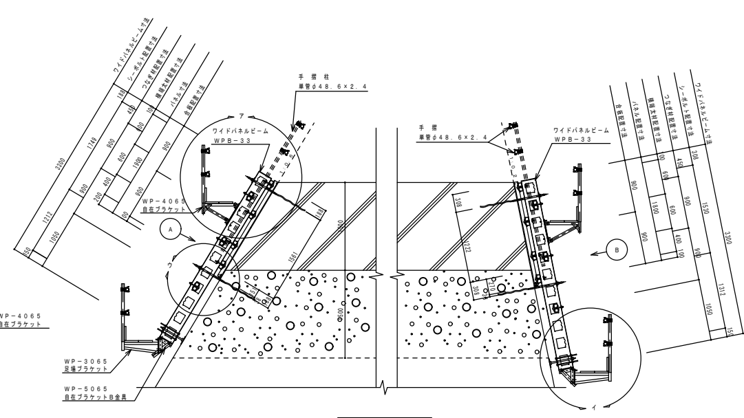
断面図 1/40
