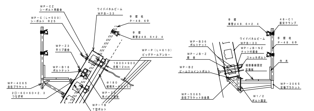
イ部 詳細図 1/20
