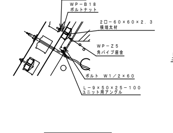
B部 詳細図 1/20
